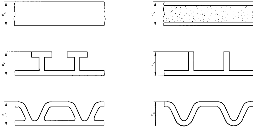
图 3 管材结构壁厚 e_c 的示例
