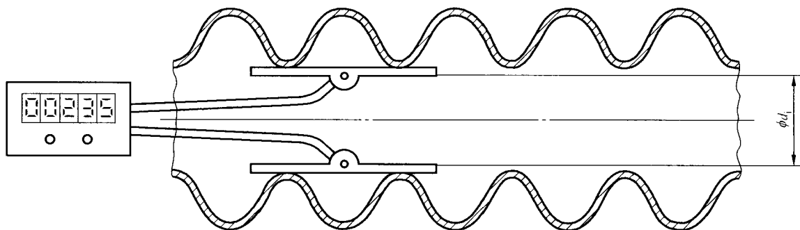
图 1 测量波纹管内径的典型装置
